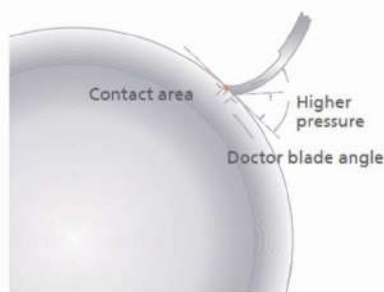
과도한 블레이드 압력
