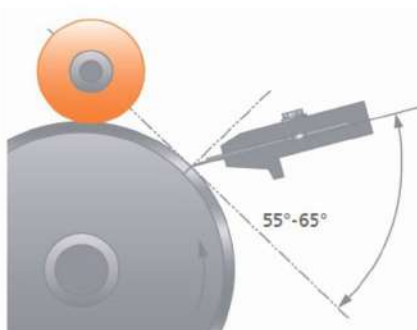
최적의 블레이드 셋팅 각도
