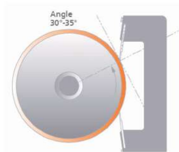
최적의 블레이드 셋팅 각도
